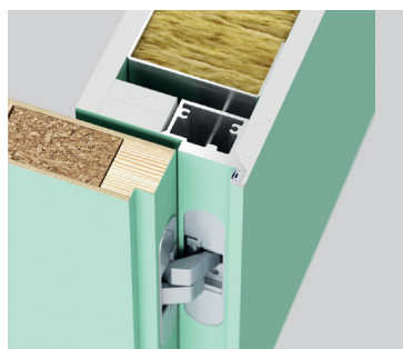
Przeciw przylga (otwierane do wewnatrz) - drzwi lewe
