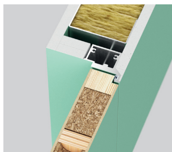
Przeciw przylga (otwierane do wewnatrz) - drzwi lewe
