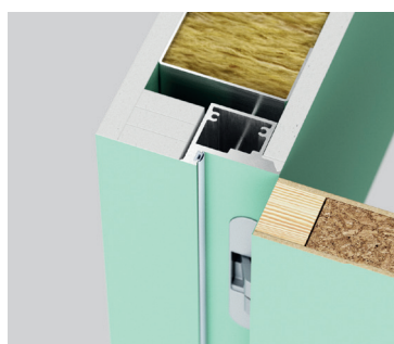
Bezprielgowe standard (otwierane na zewnatrz) - drzwi prawe
