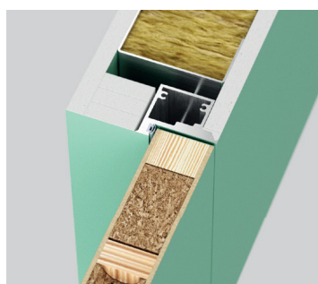
Bezprielgowe standard (otwierane na zewnatrz) - drzwi prawe
