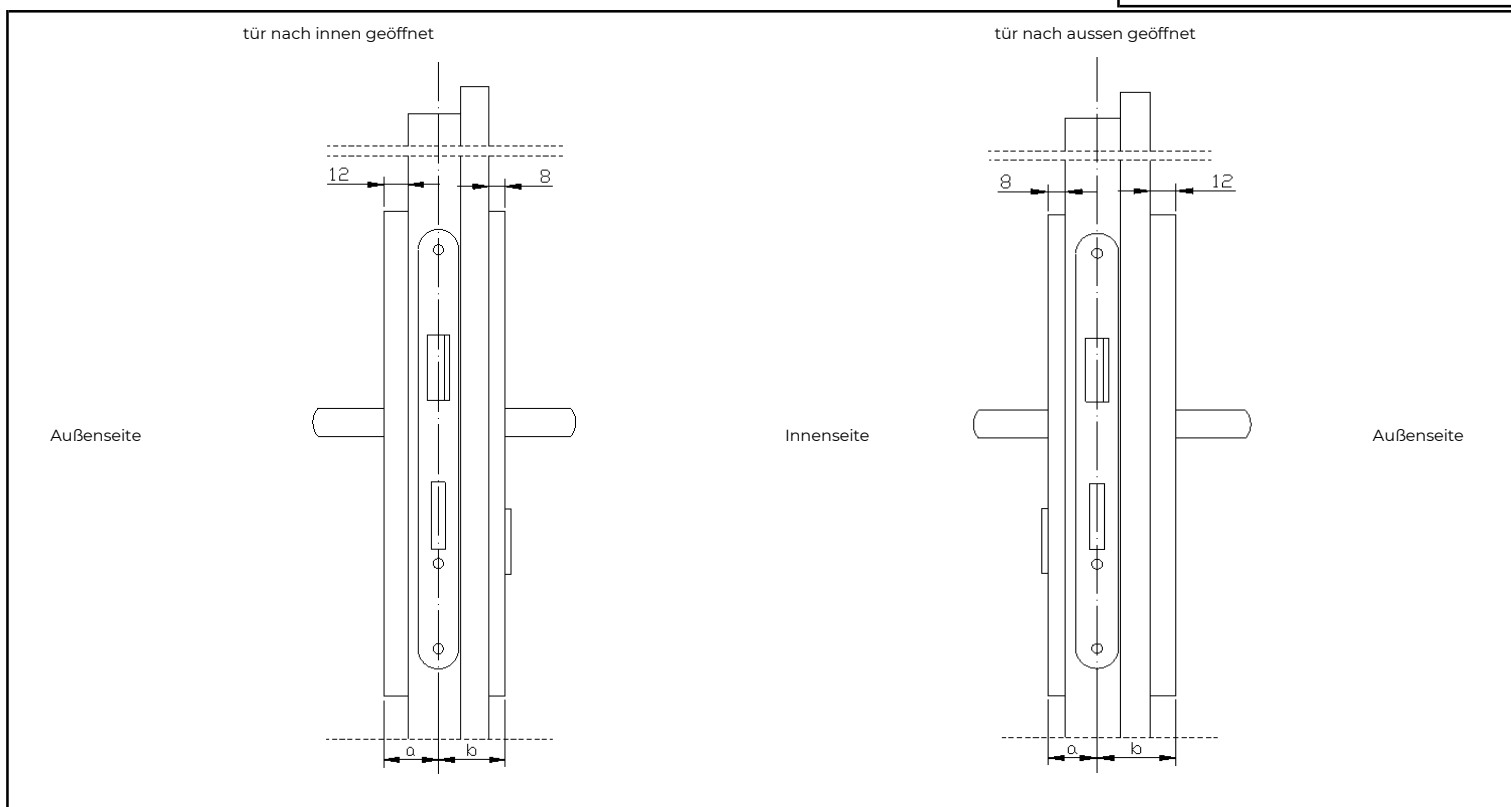
Die obige Zeichnung gilt für folgende Griffe: "Porta Opal", "Porta Granit", "Royal", "Porta Safe", "Porta Gardo**", "Porta Gardo Top**" und "Porta Gardo Oval Top**".
