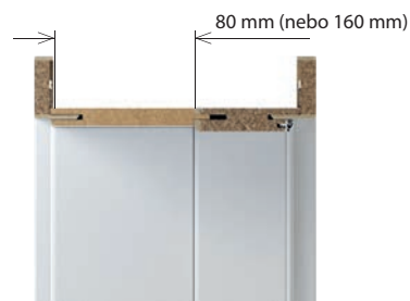
maximum zárubeň s širokým perem za příplatek
