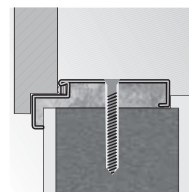
ościeżnica kąтова duża montaż na dyble
