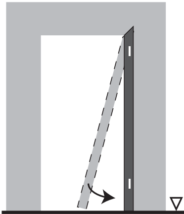
BELKA PIONOWA STRONA ZAWIASOWA
