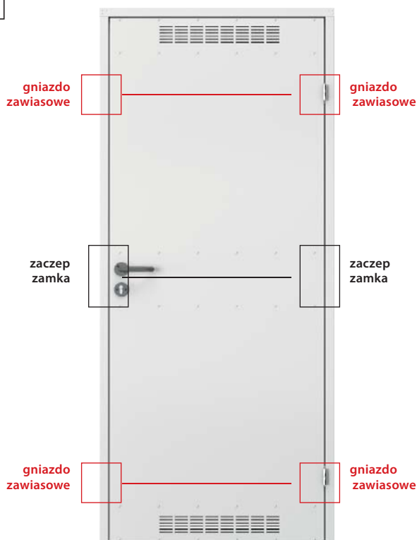
przód skrzydła
