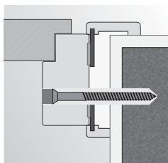
montaż na piankę i kotwy w ścianie muruwanej
