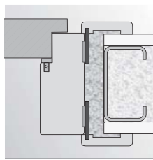
montaż na piankę w ścianie z płyty kartonowo-gipsowej
