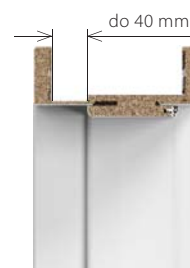
maksimum ościeżnica z szerokim piórem opcja za dopłatą do 40 mm
