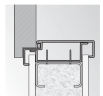
ościeżnica kąтова duża montaż na ścianie kartonowo-gipsowej
