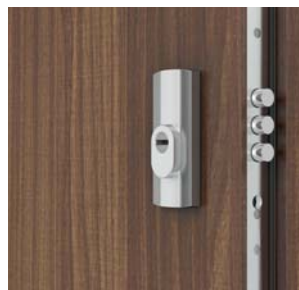
zamek listwowy wielobolcowy dostosowany pod dwie wkładki patentowe
