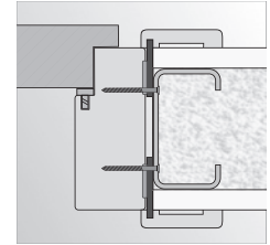
montáž na vruty do stěny ze sádkkartonu
