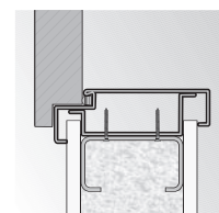
rohová zárubeň velká montáž na sádkkartonovou stěnu
