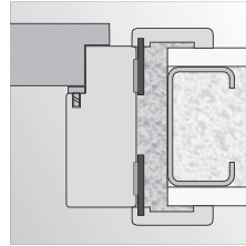
montáž na pěnu do stěny ze sádkkartonu
