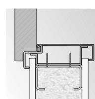
zárubňa ROHOVÁ VELKÁ montáž do sadrokartó- novej steny
