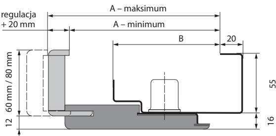
przekrój ościeżnicy PROJEKT Premium
