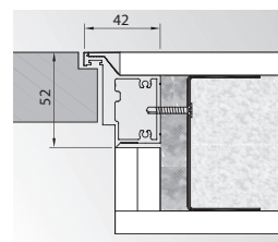
przeciwpzylgła (otwierane do wewnątrz)
