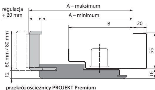
ościeżnica PROJEKT Premium
