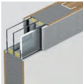
Dwukomorowe przeszklenie antywlamaniowe klasy P4 i ramka ze stali nierdzewnej
