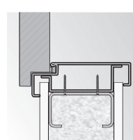
ościeznica Kątowa DUŻA montaż na ścianie kartonowo-gipsowej
