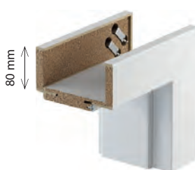
profil ościeżnicy – szeroka listwa 80 mm
