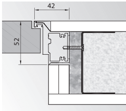
przeciwpzylga (otwierane do wewnątrz)
