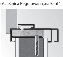
ościeznica Regulowana „na kant”
