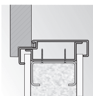
ościeznica Kątowa DUŻA montaż na ścianie kartonowo-gipsowej
