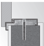
ościeznica Kątowa DUŻA montaż na dyble
