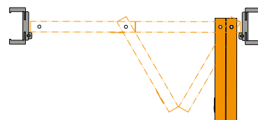
SPÔSOB OTVÁRANIA DVERÍ (pohľad zhora)
