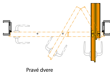
SPÔSOB OTVÁRANIA DVERÍ (pohľad zhora)
