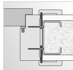
skrutkovanie do steny zo sadrokartónu
