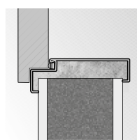
inštalácia bez dodatočných kotviacich prvkov
