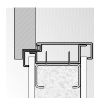
zárubňa rohová VEĽKÁ montáž na SDK stenu
