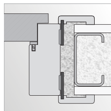
montáž na penu do steny ze sádrokartonu
