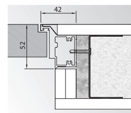
Reverzní podrážka (otevírané dovnitř)
