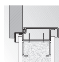
rohová záruben velká montáž na sádrokartonovou stenu
