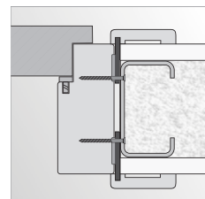
montáž na vruty do steny ze sádrokartonu
