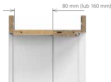
wersja z panelem regulującym (80, 160 mm)
