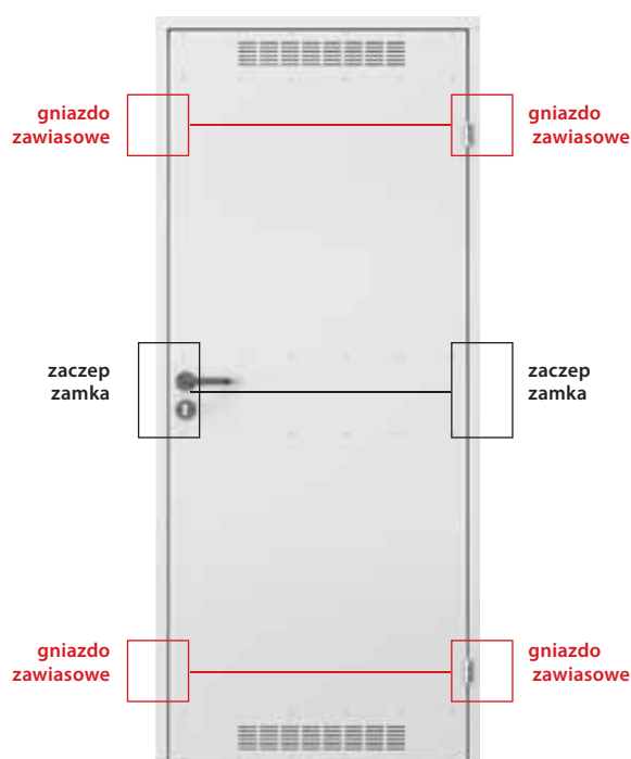
przód skrzydła
