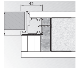
Porta HIDE ellentétes éllel (befelé nyíló)
