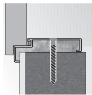
nagy saroktok dűbeles beépítése
