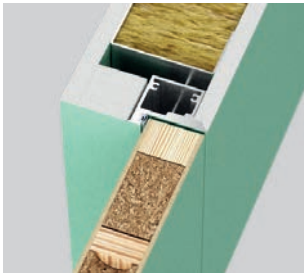
Falc nélküli standard (kifelé nyíló) – jobbos ajtó
