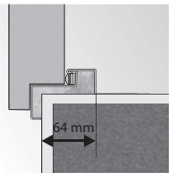
kis saroktok
