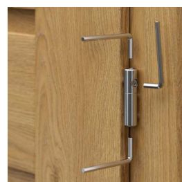
a PORTA KONCEPT 3D állítható ajtópántjainak beállítása
