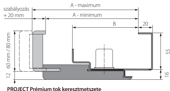
PROJECT Prémium tok keresztmetszete
