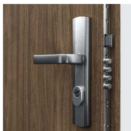
többpontos szalagzár két cylinderbetéhez
