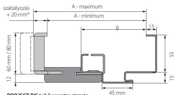
PROJECT BIS tok keresztmetszete
