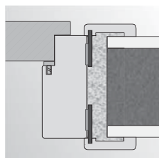
montaż na piankę w ścianie murowanej
