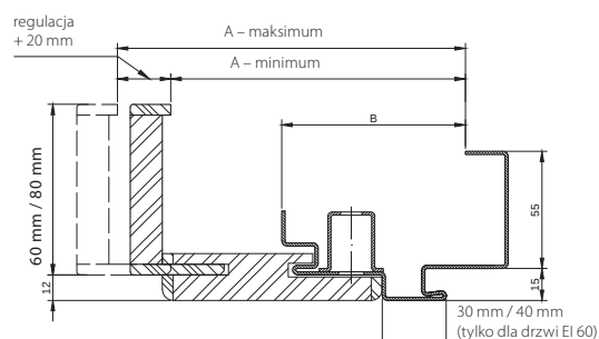
przekrój ościeżnicy PROJEKT
