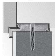
ościeżnica Kątowa DUŻA montaż na dyble
