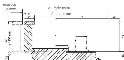
przekrój ościeżnicy PROJEKT Premium
