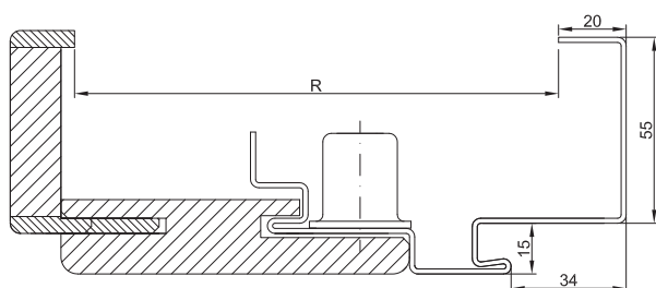
Ościeżnica Regulowana Projekt
