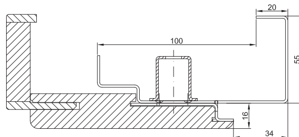
Ościeżnica Regulowana Projekt Premium
