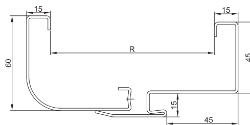
Ościeżnica Regulowana z R do drzwi bezprzylgowych
