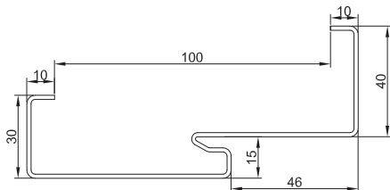
Ościeżnica p.poż. dostosowana do drzwi drewnianych EI60 marki PORTA
