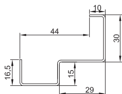
Ościeżnica Kątowa Mała bez zagięcia pod uszczelkę
