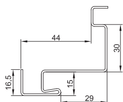
Ościeżnica Kątowa Mała z zagięciem oddzielającym
