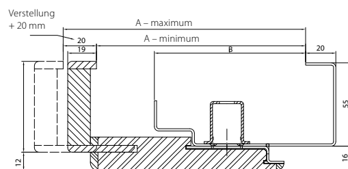
PROJECT Premium zargenquerschnitt
