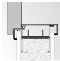
Montage an Gipskartonwänden große Eckzarge
