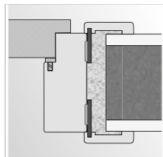
Montage mit Schaum in Mauerwand
