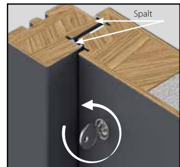
NACH dem Schließen ~ 3 mm
