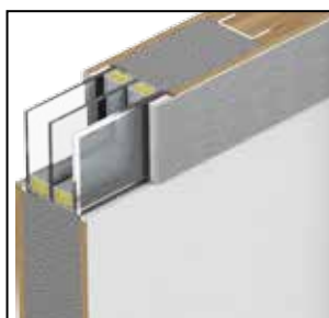
Dreischeiben-Verglasung, einbruchhemmend, Klasse P4 und Rahmen aus rostfreiem Stahl
