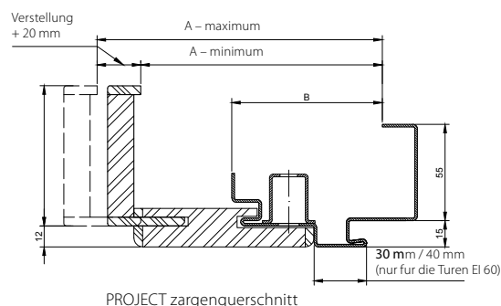
PROJECT zargenquerschnitt
