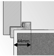
Eckzarge Klein
