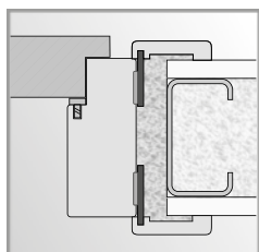
Montage mit Schaum in Gipskartonwänden
