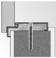
Montage mit Dübeln große Eckzarge
