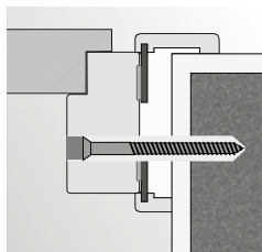
Montage mit Schaum und Anker in Mauerwand
