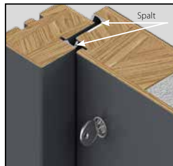
VOR dem Schließen ~ 5 mm
