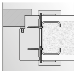
Montage mit Schraube in Gipskartonwänden
