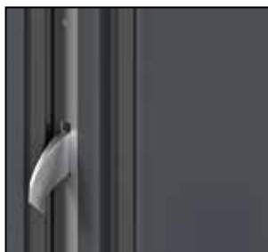
Mehrpunktverriegelung mit Spanmechanismus Winkhaus STV • Schmiedeeisen Haken • Schließblech-Regulierung
